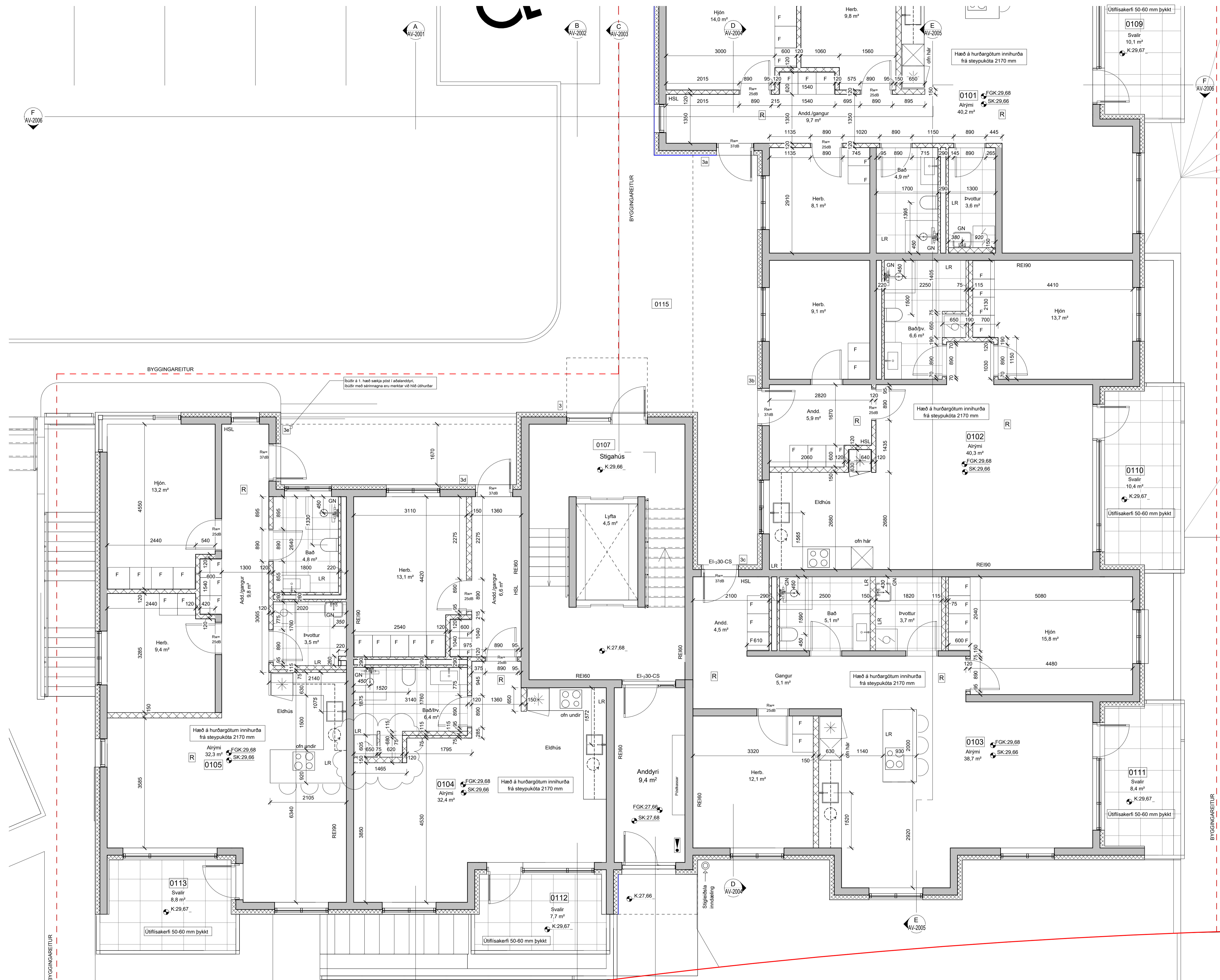
1.HÆÐ - VERKTEIKNING - C mkb: 1 : 50
